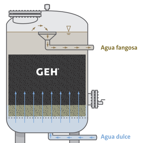
Fig. 3: Retrolavado de instalación
