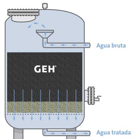
Fig. 5: Funcionamiento del adsorbedor
