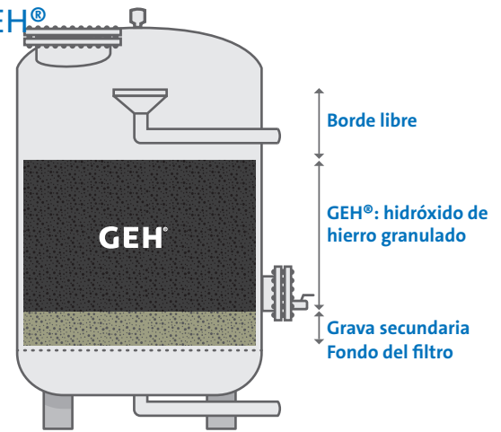
Fig. 1: Diseño básico de las unidades de adsorción de GEH®
